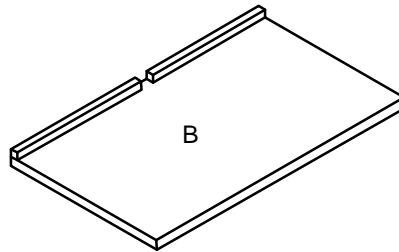
Bx3 576x340x33 mm
